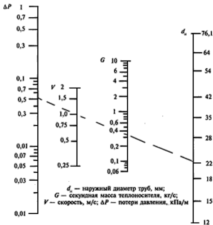
Рисунок В.2 - Система отопления
