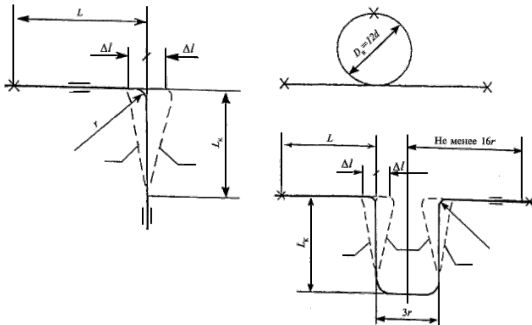
Рисунок Д.1 - Расчетные схемы гнутых компенсаторов*
