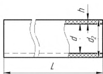
а) труба с присоединительными частями без утолщений
