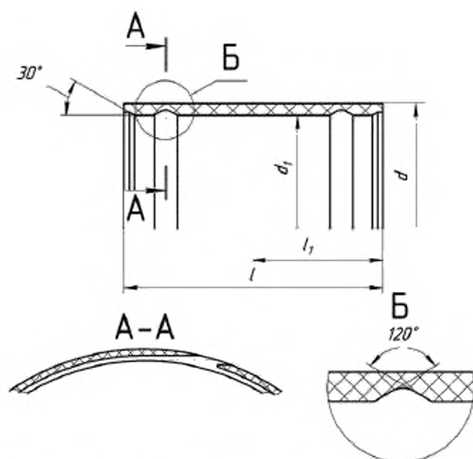
Рисунок 9 – Муфта типа МКЛ для соединения «КЛ»
