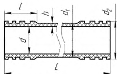
б) труба с присоединительными частями и утолщениями
