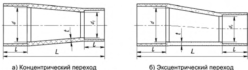
Рисунок 17 – Основные размеры перехода
