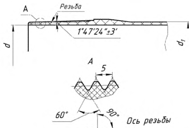
Рисунок 5 – Резьбовая концевая часть под соединение «РКН»
