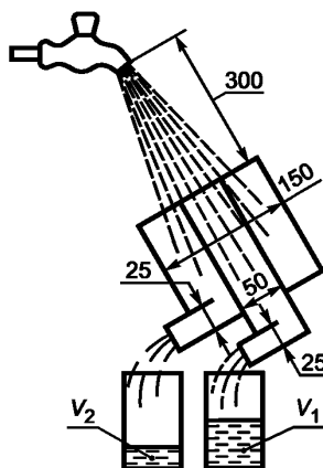
Рисунок 1 — Схема определения компактности струи
