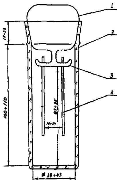
Рисунок 1. Схема лабораторной установки:
