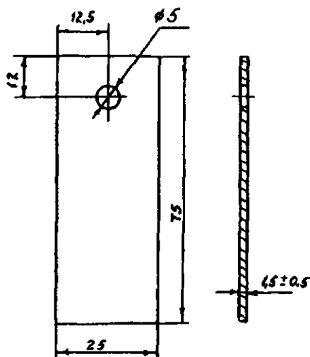
Рисунок 2. Эталонная металлическая пластина
