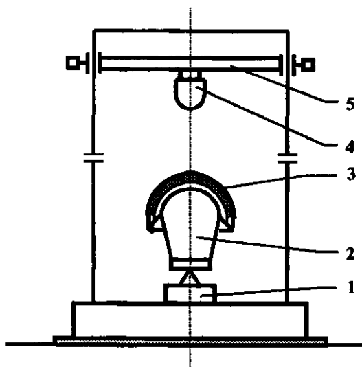
Рис. 1. Принципиальная схема стенда ударного: 1 - силоизмерительный датчик; 2 - муляж головы; 3 - каска; 4 - ударник; 5 - каретка
