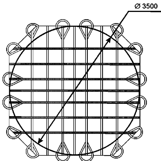
Рисунок 1 — Конструкция ПСН
