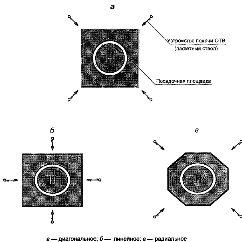
Рисунок А.1 — Схемы размещения стационарных лафетных стволов
