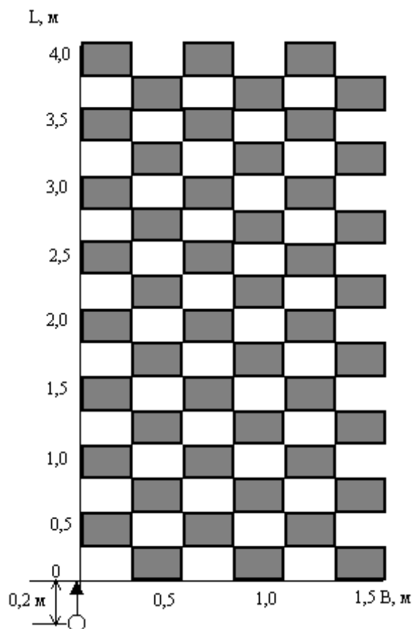
Рис. 3. Схема расположения мерных банок при испытании водяных оросителей типа Г и Гв:
