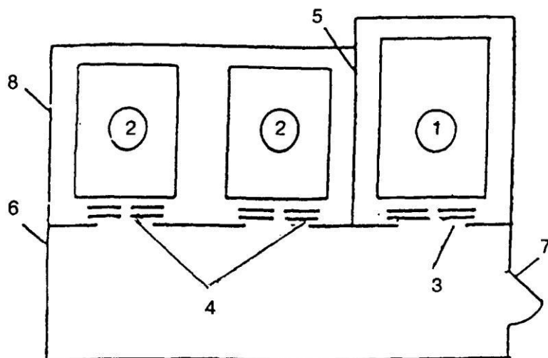
Рисунок 1 — Размещение в общей шахте с другими пассажирскими лифтами
