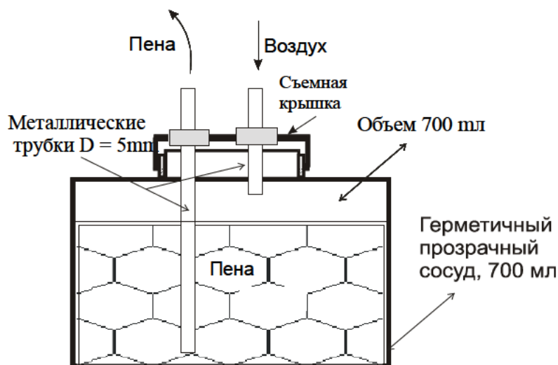
Рис. 3. Схема конструкции разъемного герметичного контейнера для контроля массы пены, израсходованной на тушение
