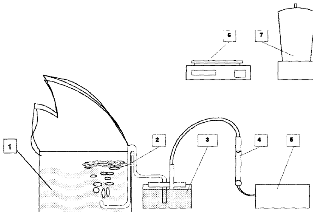
Рис. 1. Схема стендовой установки для определения времени тушения:
